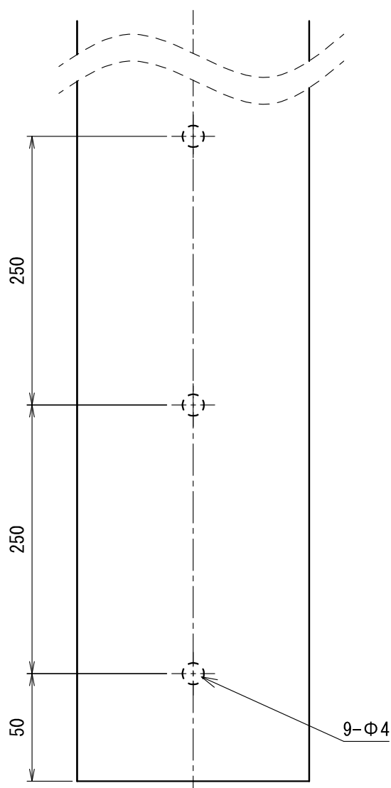
ビス取付穴ピッチ
